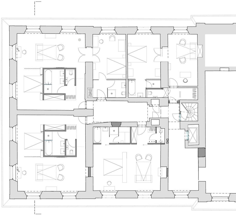
Grundriss OG3
