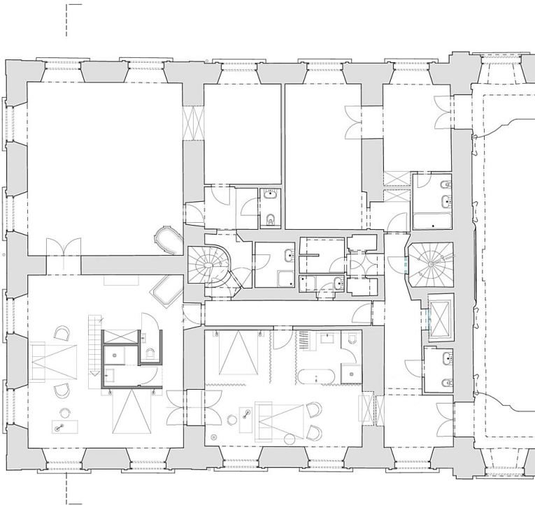
Grundriss OG2
