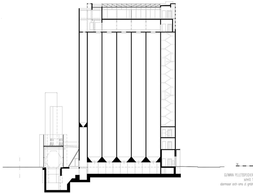
Schnitt 1
