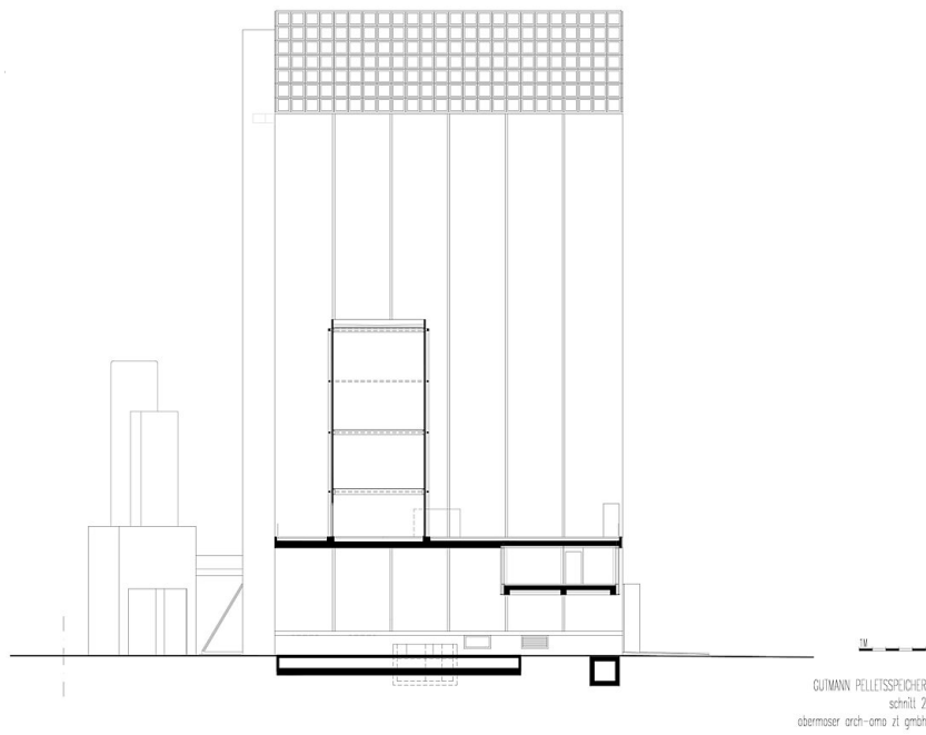
Schnitt 2
