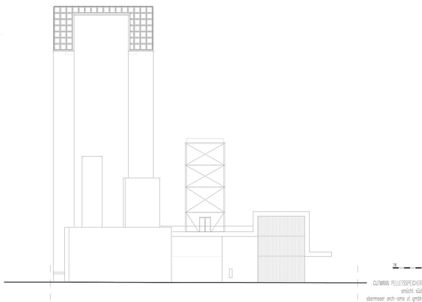
Ansicht Süd
