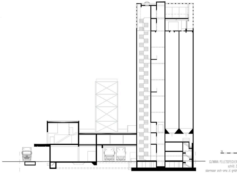
Schnitt 3
