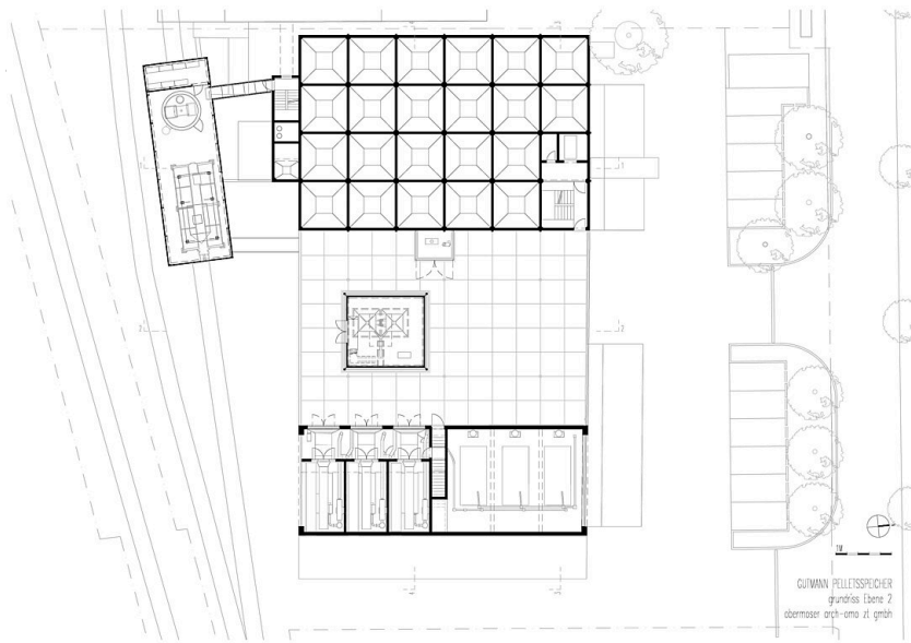
Grundriss Ebene 2
