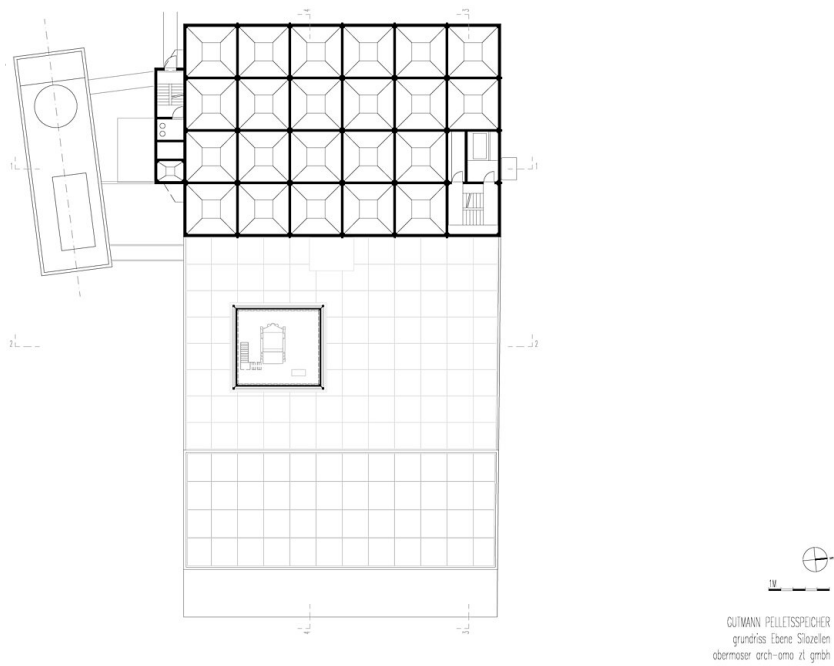
Grundriss Ebene Silo
