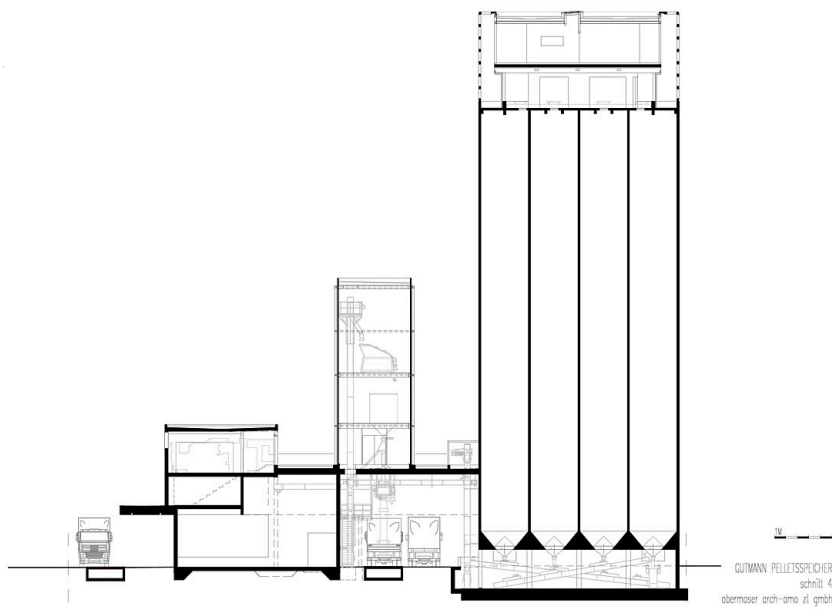
Schnitt 4
