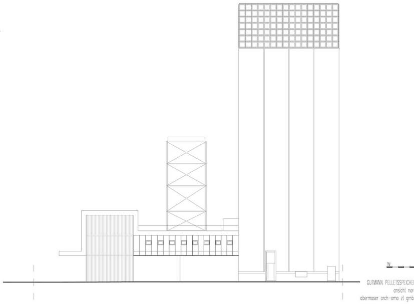
Ansicht Nord
