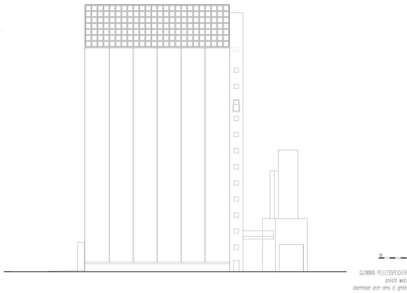
Ansicht West
