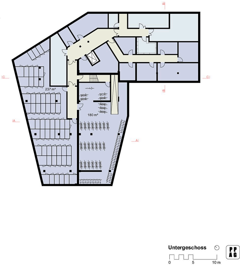
Grundriss UG
