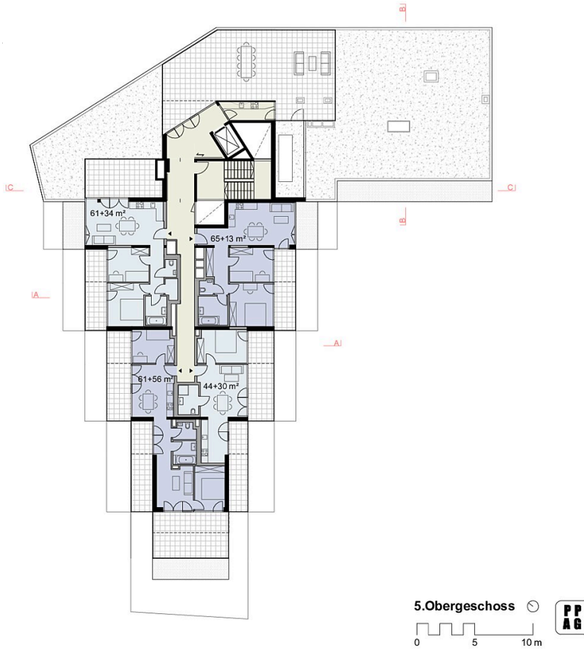
Grundriss OG5
