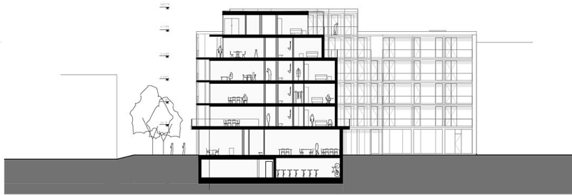
Schnitt A-A
