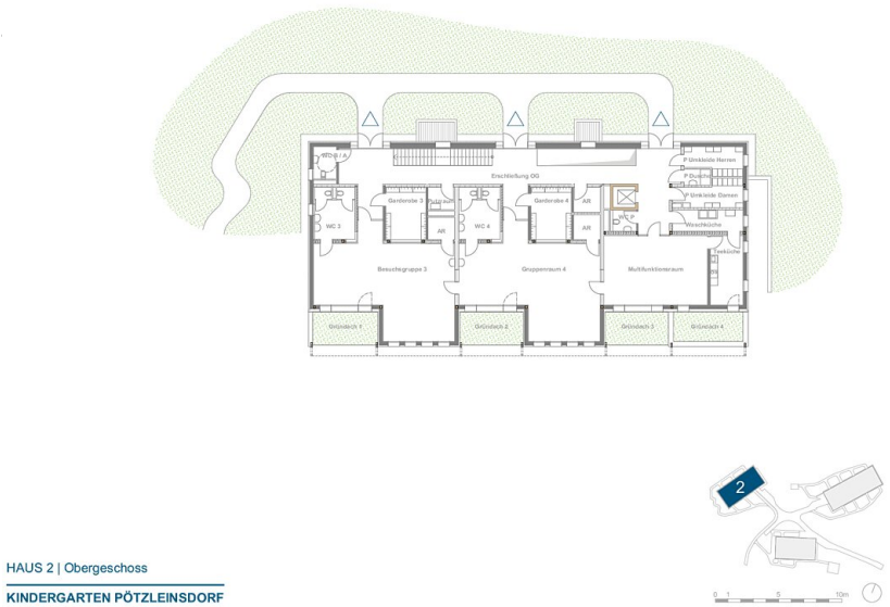
Haus 2 Grundriss OG
