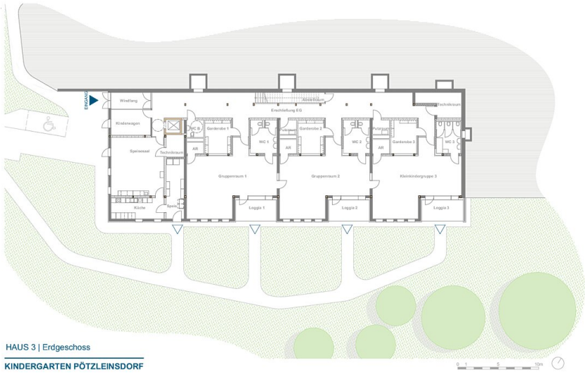
Haus 3 Grundriss EG
