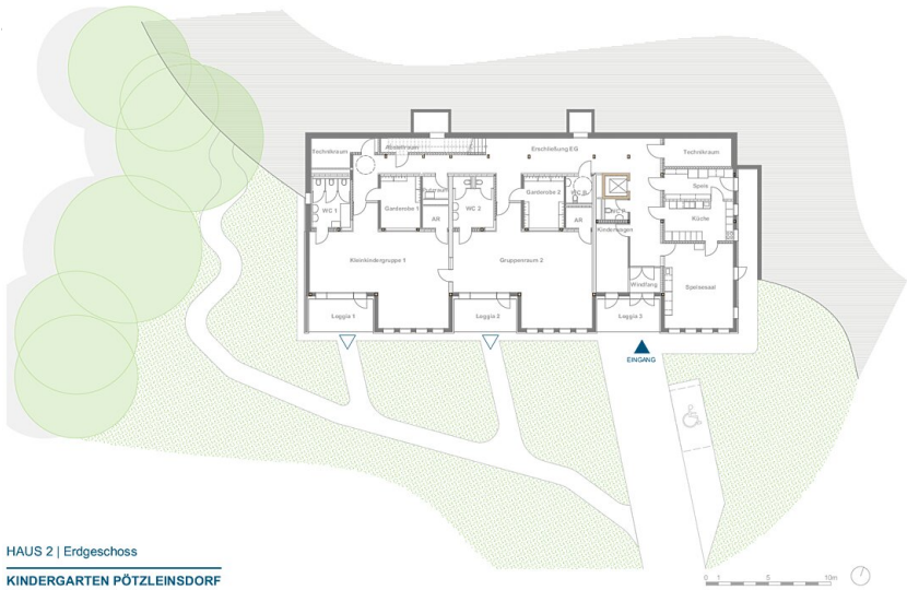
Haus 2 Grundriss EG
