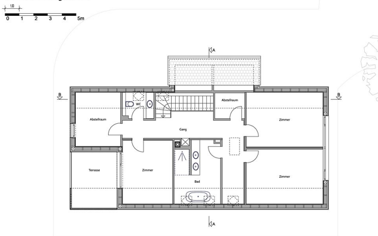
Grundriss Obergeschoß
