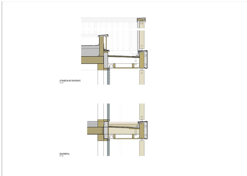
Fassadenschnitte
