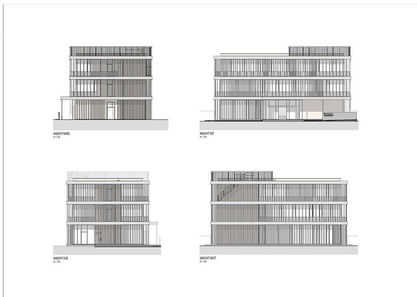
Ansichten
