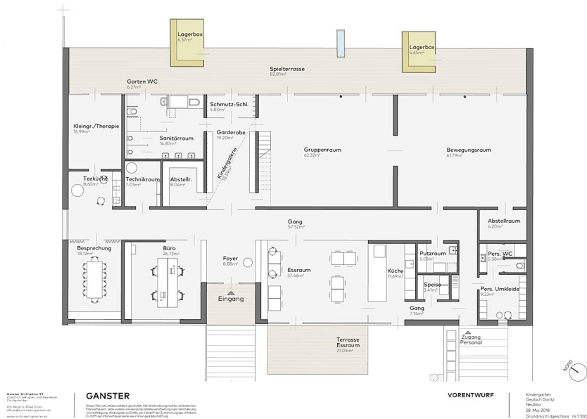
Grundriss
