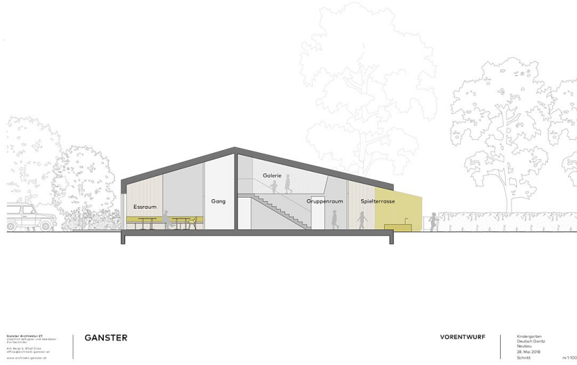
Schnitt 1
