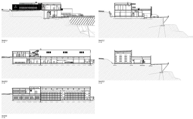
Schnitte
