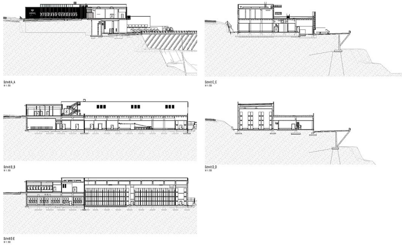
Schnitt E 1:100
