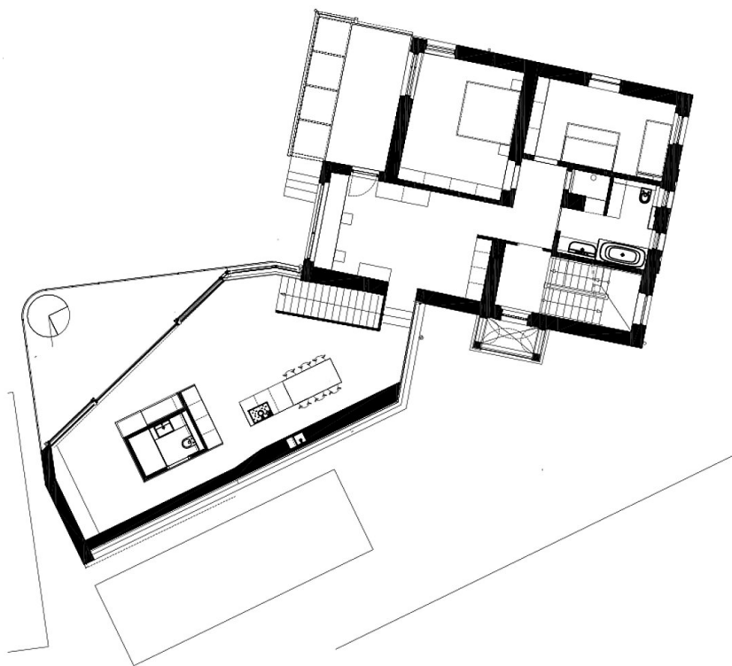
Grundriss OG
