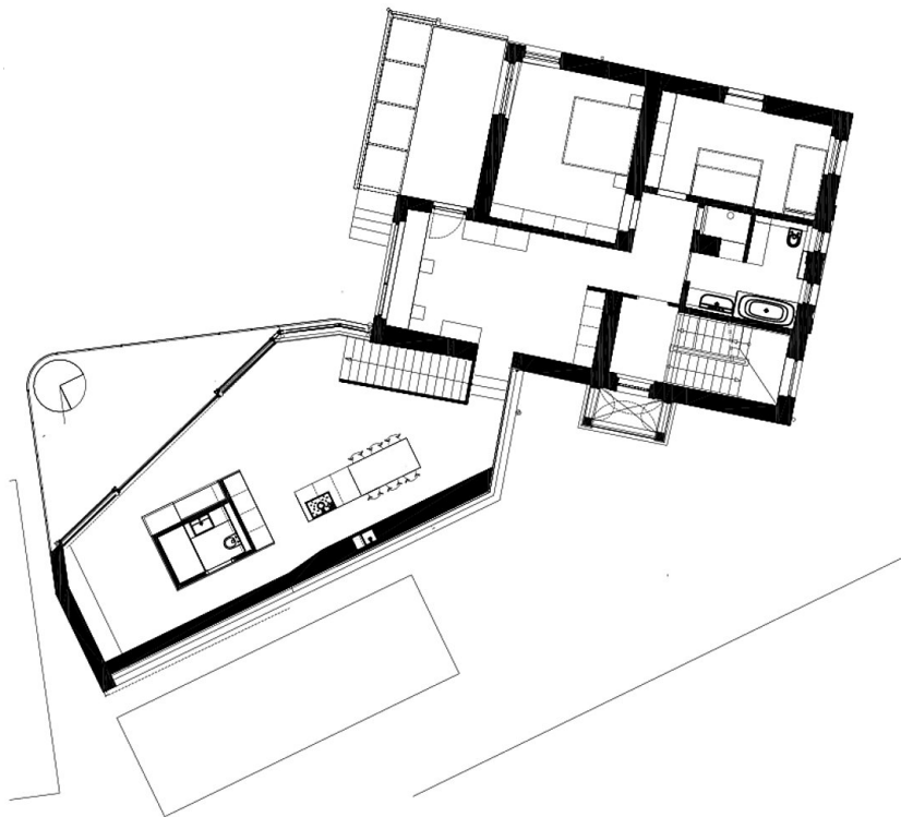
Grundriss OG
