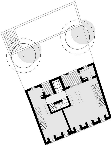
Grundriss OG3
