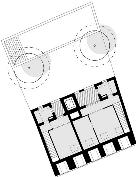
Grundriss DG
