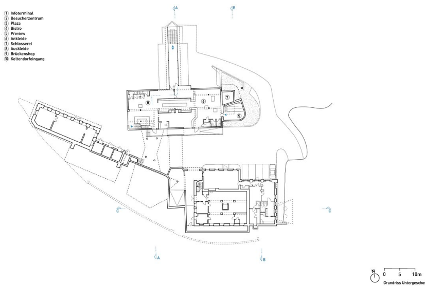
Grundriss UG
