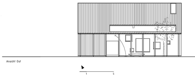
Ansicht Ost
