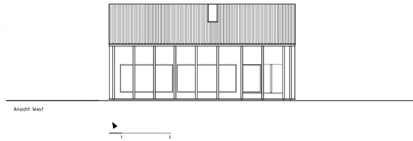
Ansicht West
