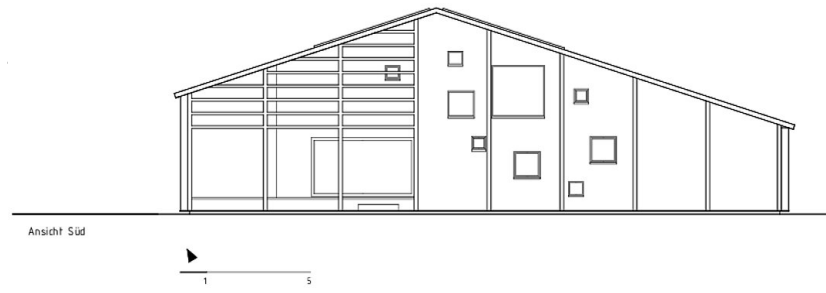
Ansicht Süd
