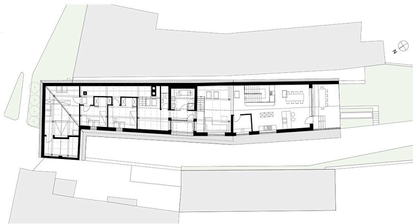
Grundriss DG
