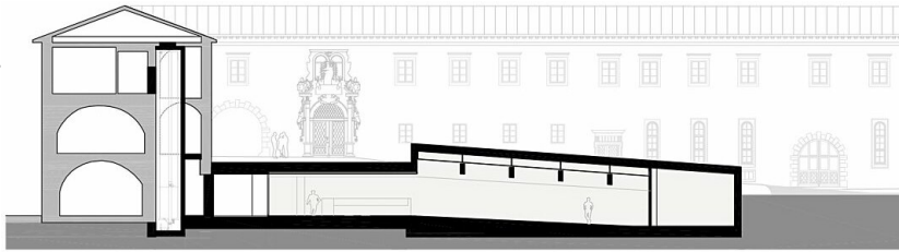
Schnitt 1
