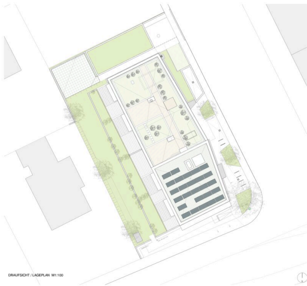
DRAUFSICHT / LAGEPLAN M1:100
