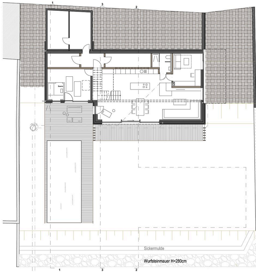
GRUNDRISS GARTENGESCHOSS
