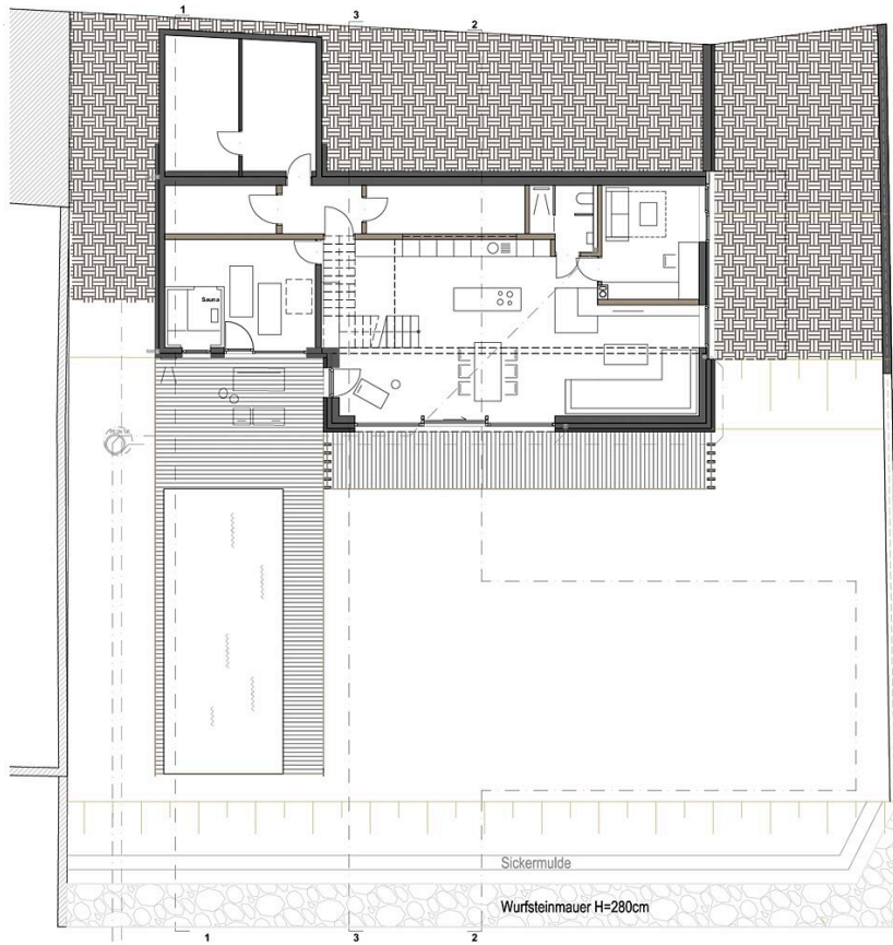
GRUNDRISS GARTENGESCHOSS
