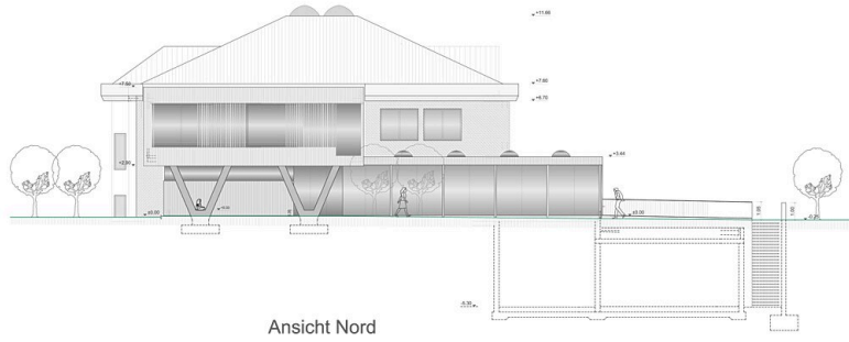
Ansicht Nord
