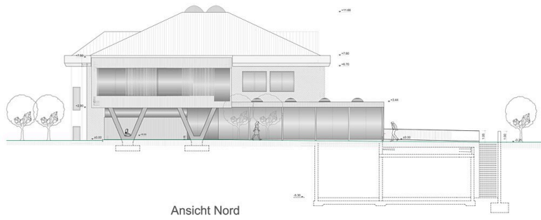
Ansicht Nord
