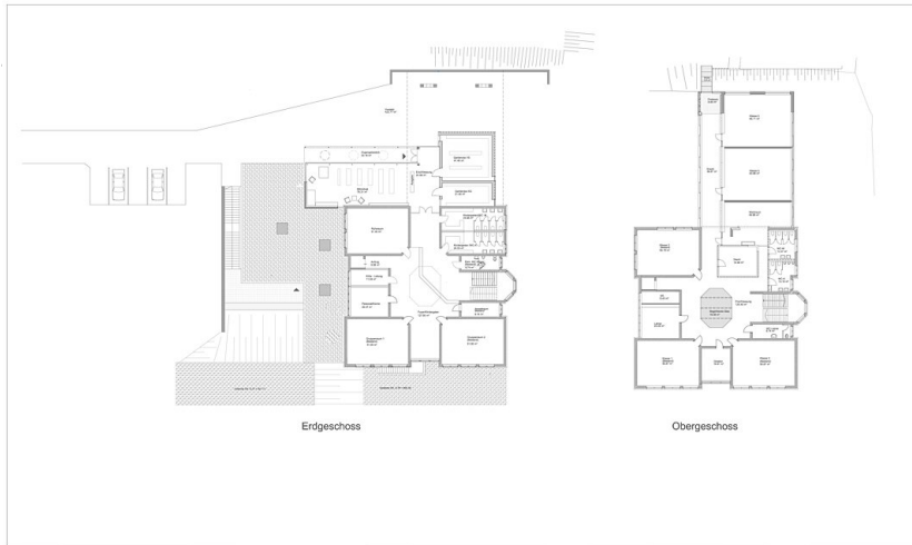
Grundrisse EG, OG
