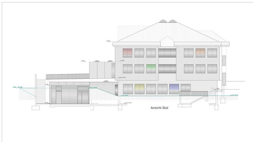
Ansicht Süd
