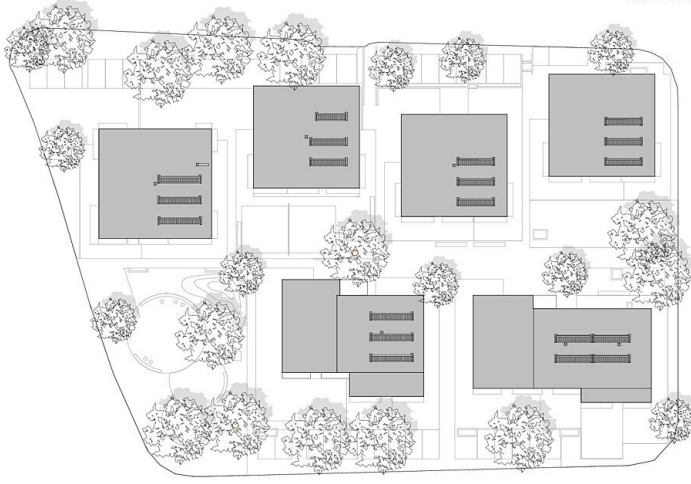
Dachdraufsicht 1:500
