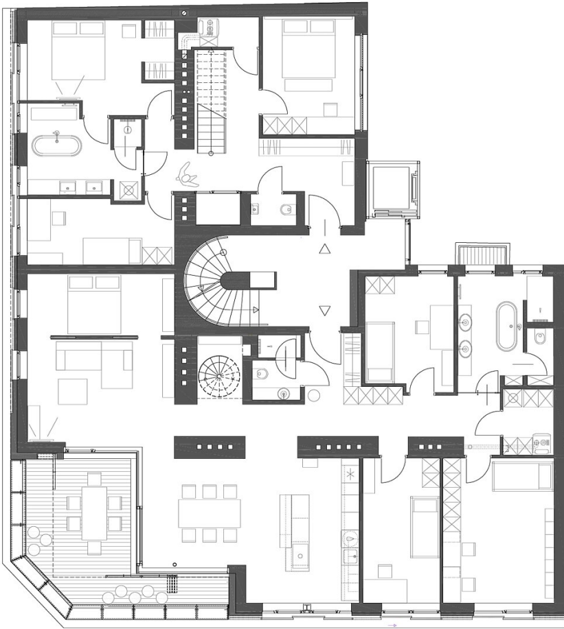
Grundriss DG1
