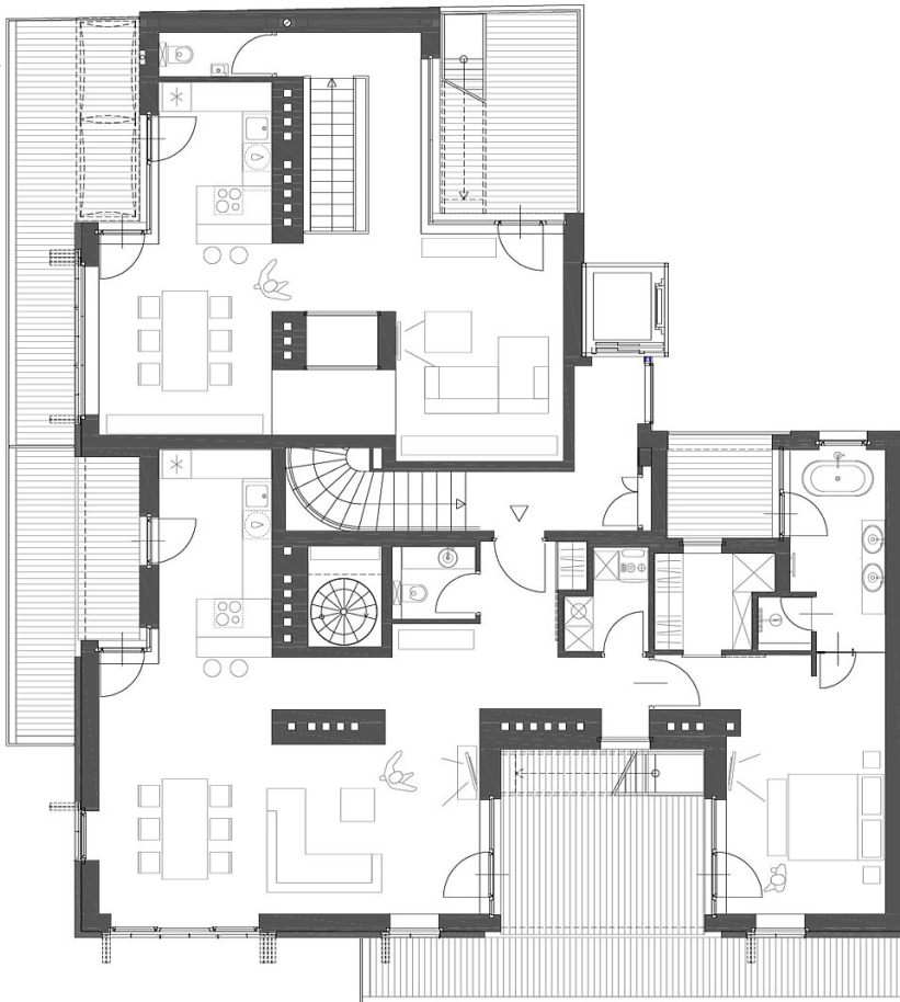
Grundriss DG2
