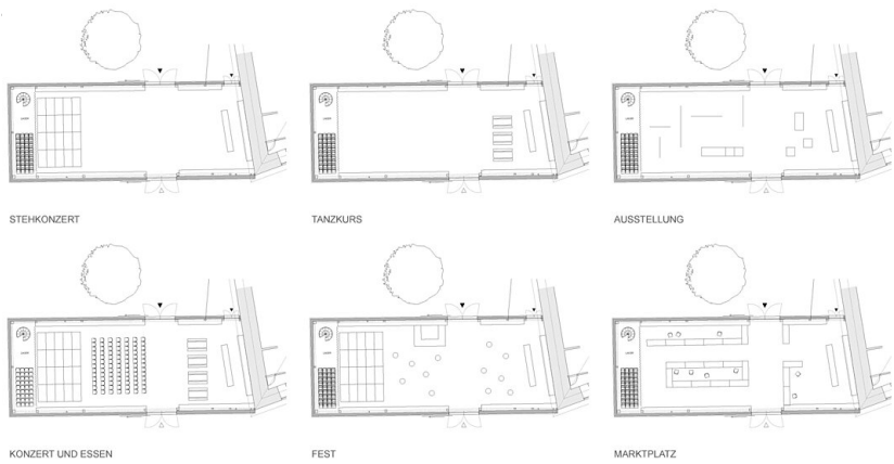
BESPIELUNGSARTEN M 1:250
