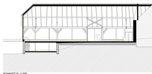
SCHNITT D 1:200
