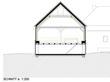
SCHNITT A 1:200
