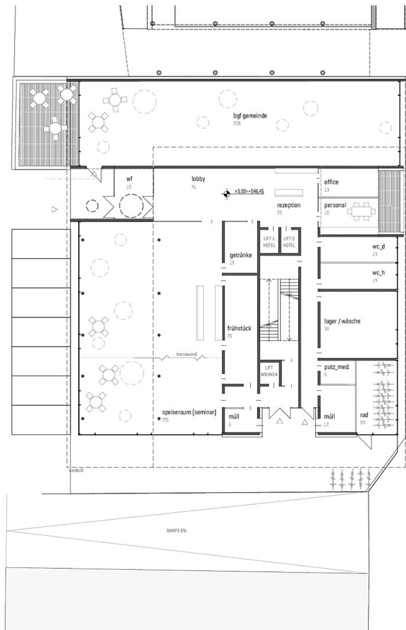
Grundriss EG
