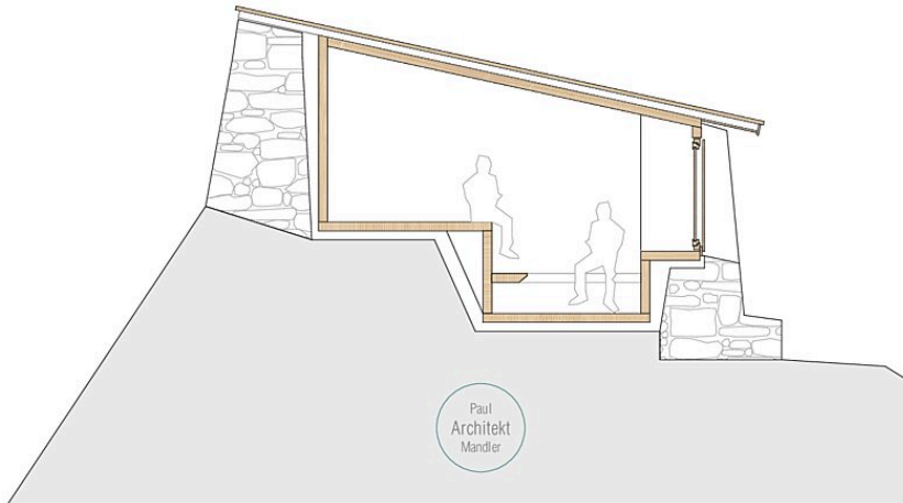
Grundriss, Schnitt
