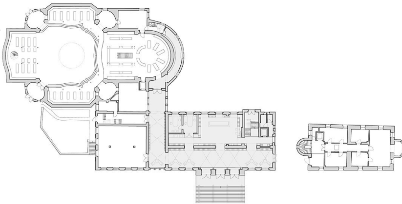
Grundriss EG
