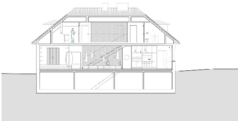
Schnitt 2
