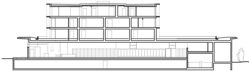
Schnitt
