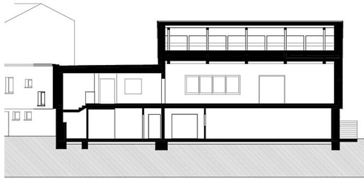
Schnitt A-A
