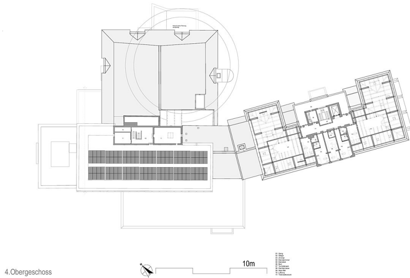
Grundriss OG4
