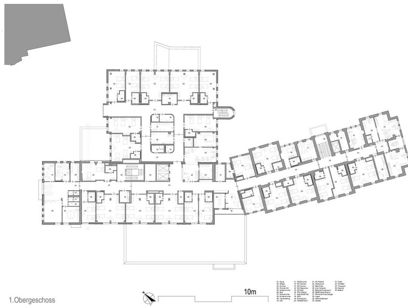
1.Obergeschoss
