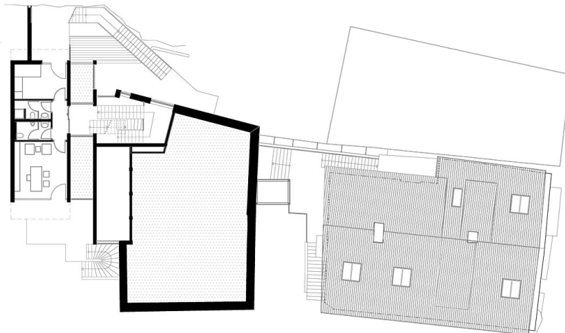
Grundriss OG3
