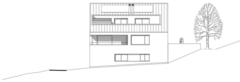
ANSICHT SÜDEN
