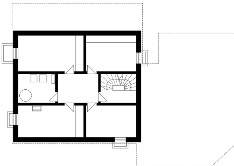
Grundriss KG
