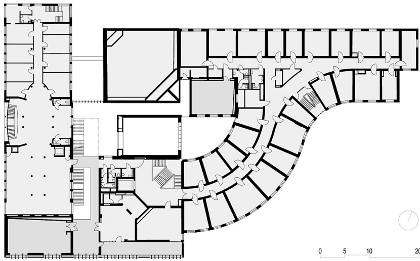
Grundriss OG1
