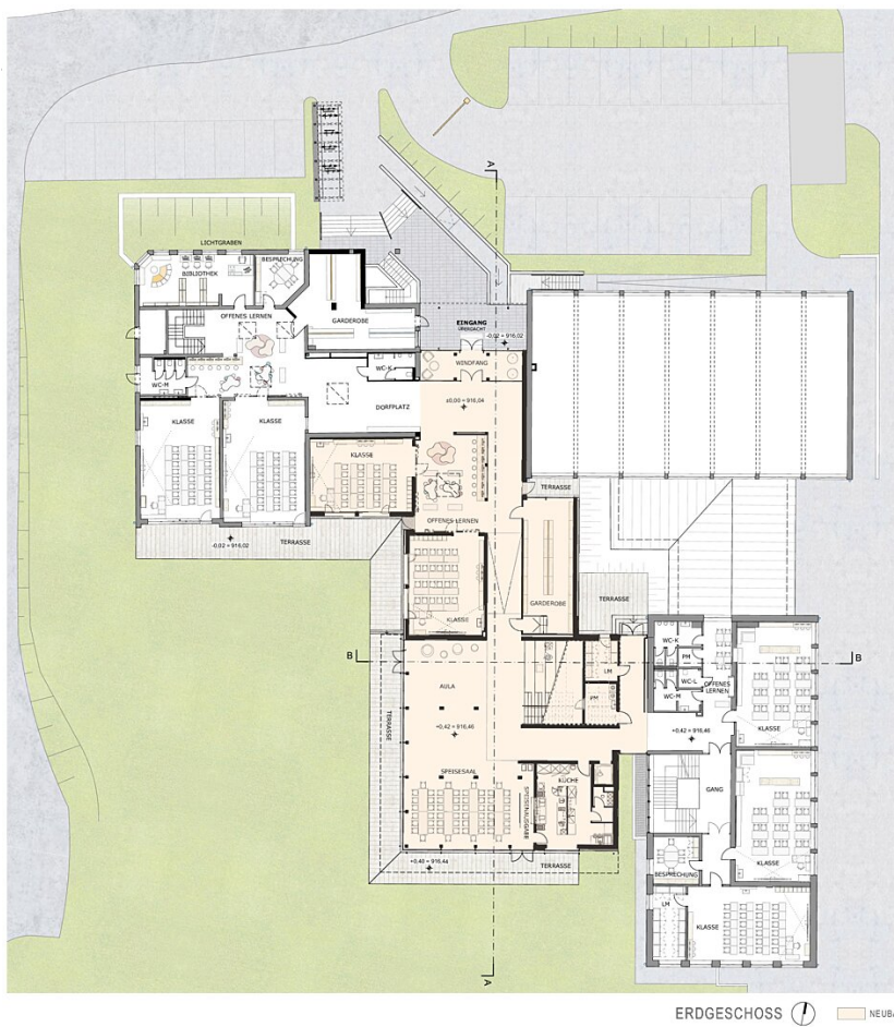
Grundriss EG
