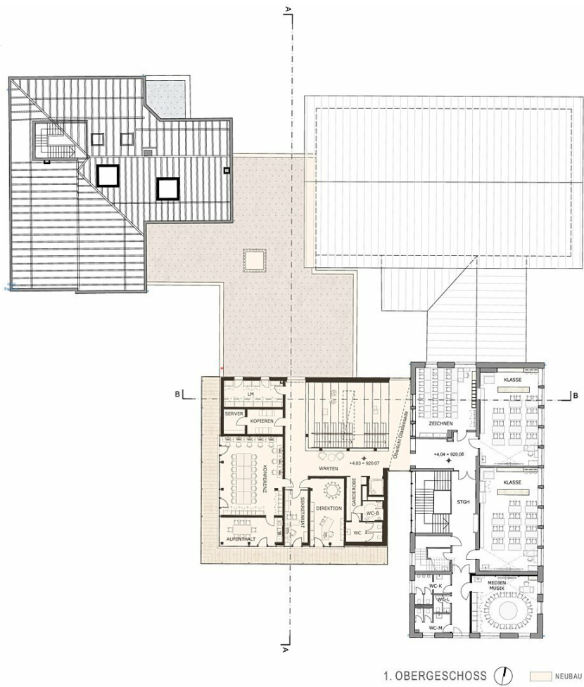
Grundriss OG
