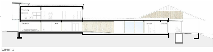
Schnitt A
