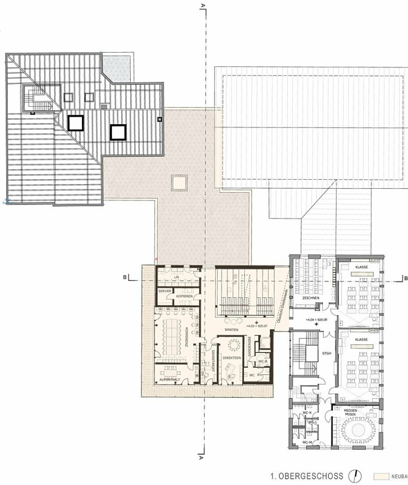
Grundriss OG
