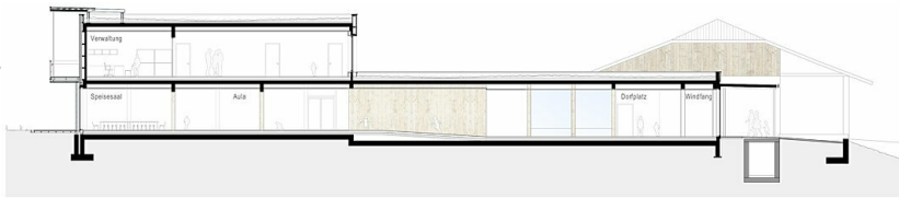
SCHNITT - A
