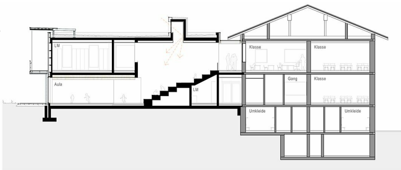
SCHNITT - B
