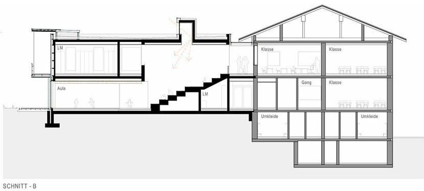
Schnitt B
