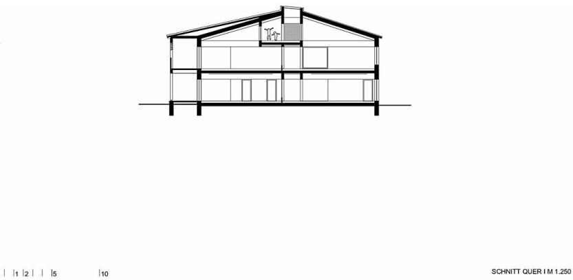
Querschnitt
