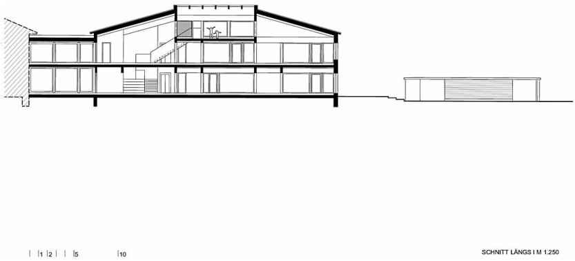
Längsschnitt
