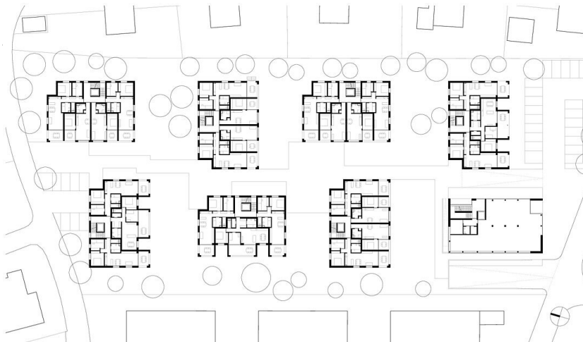
Grundrisse OG1
