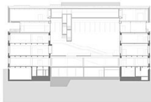
LANGSCHNITT
