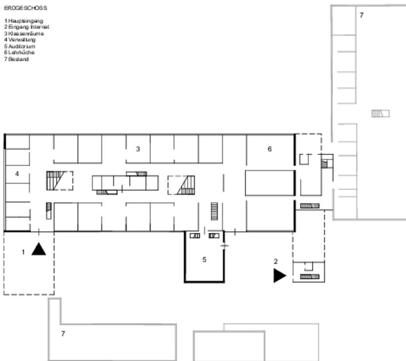
Grundriss EG
