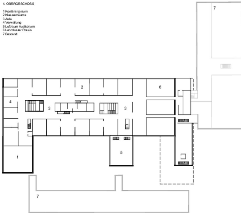
Grundriss OG1
