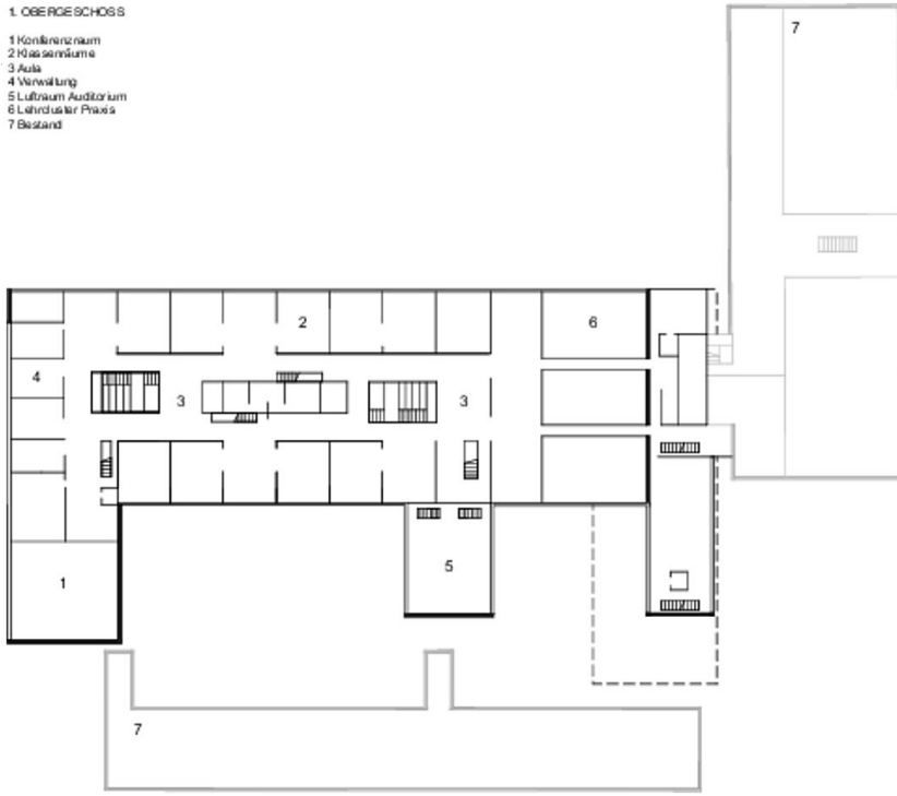
Grundriss OG1
