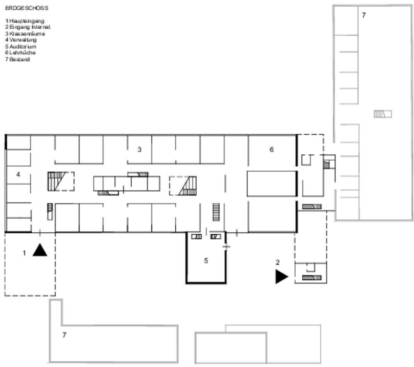
Grundriss EG
