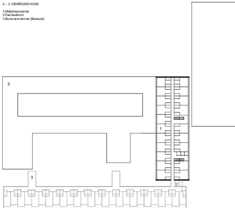
Grundriss OG3
