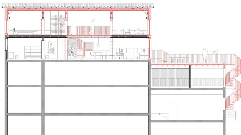
Schnitt 4
