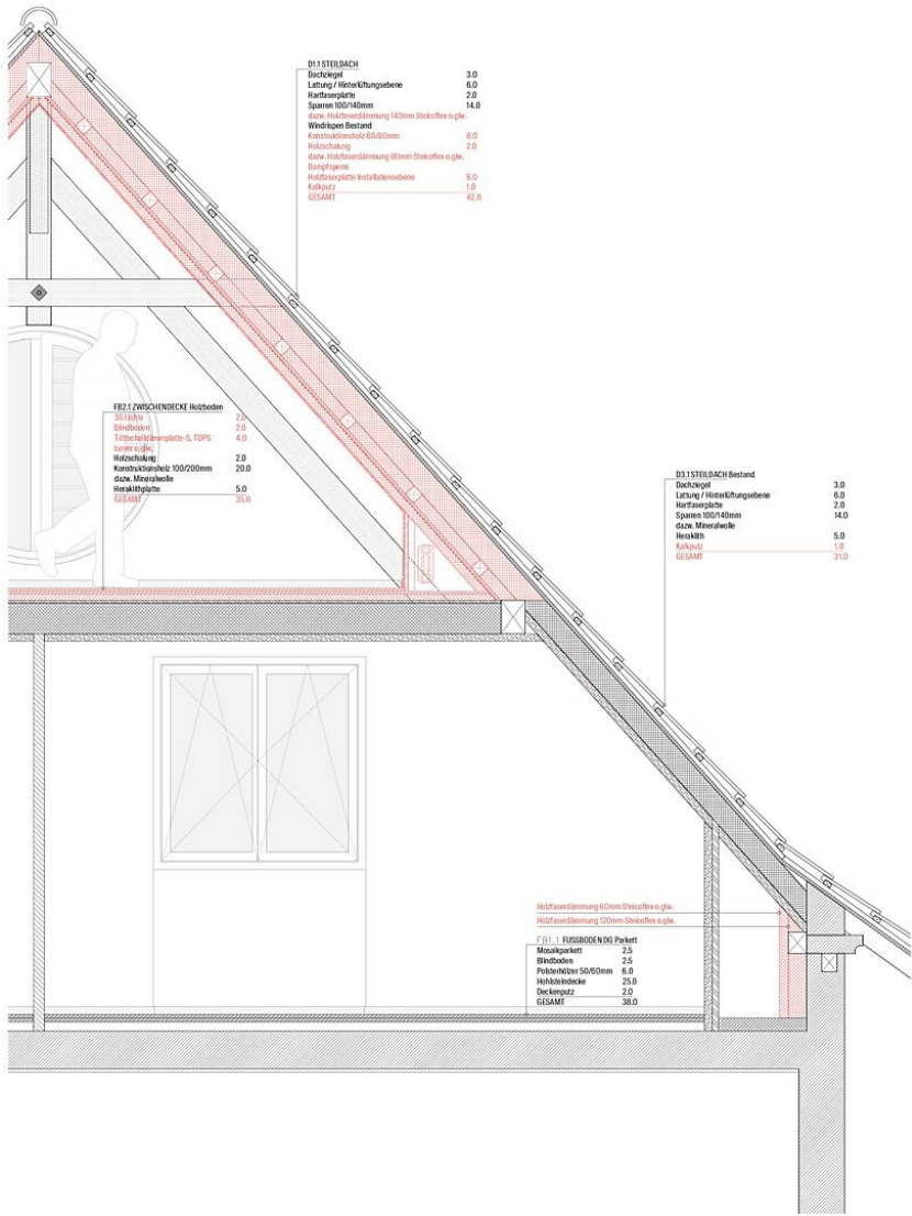
Detail 1a
