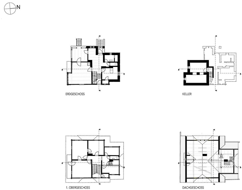
Grundrisse Bestand
