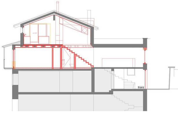
Längsschnitt Umbau
