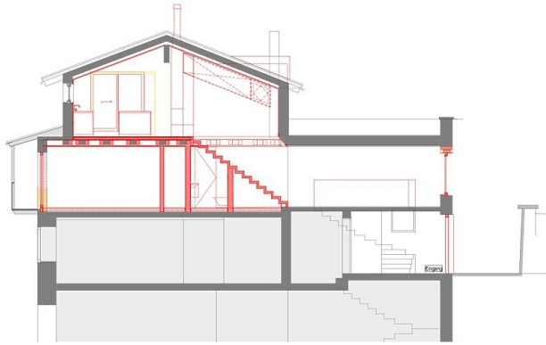
Längsschnitt Umbau
