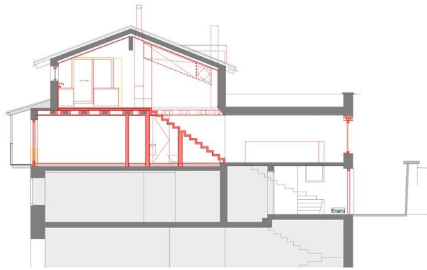
Längsschnitt Umbau
