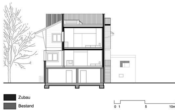
QUERSCHNITT 2
