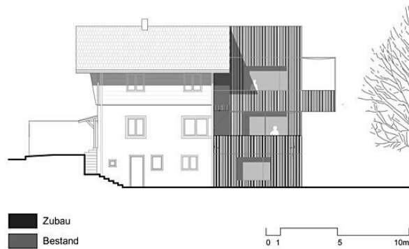
ANSICHT WEST
