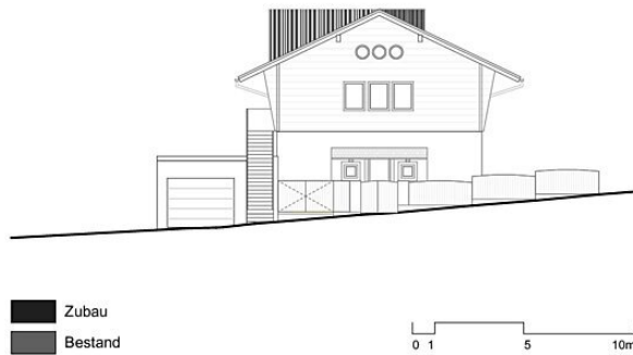
ANSICHT NORD
