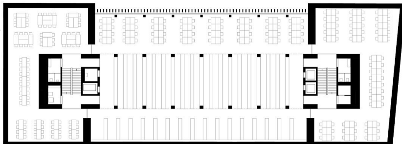
Grundriss OG2 & OG4
