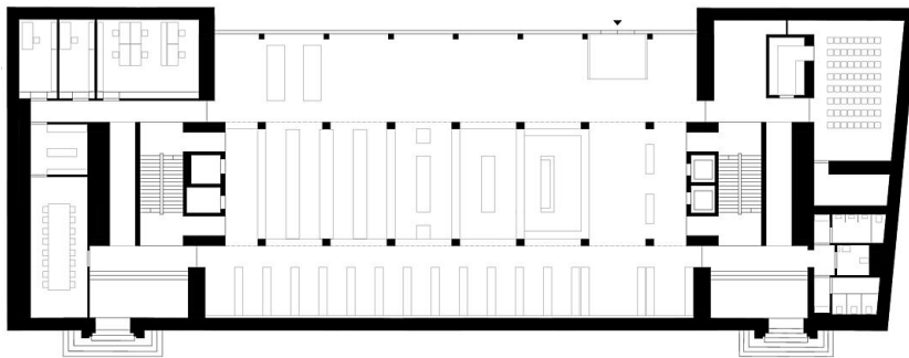
Grundriss EG
