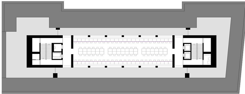
Grundriss OG7
