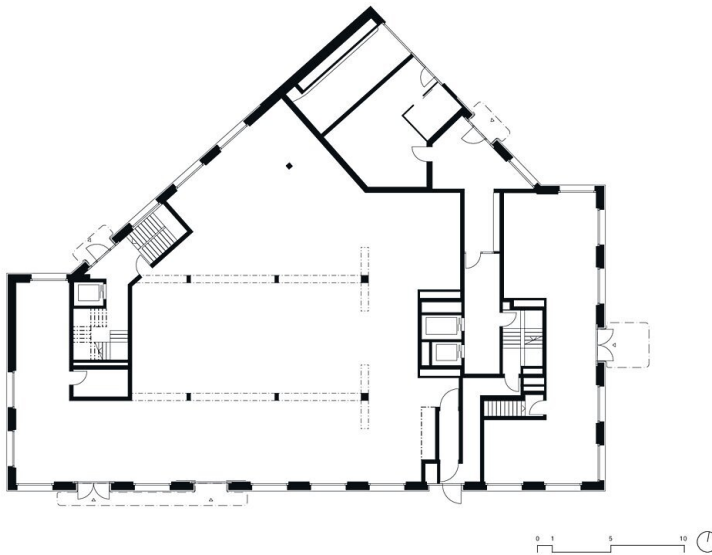
Grundriss EG
