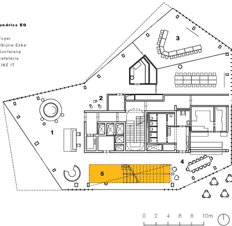
Grundriss EG
