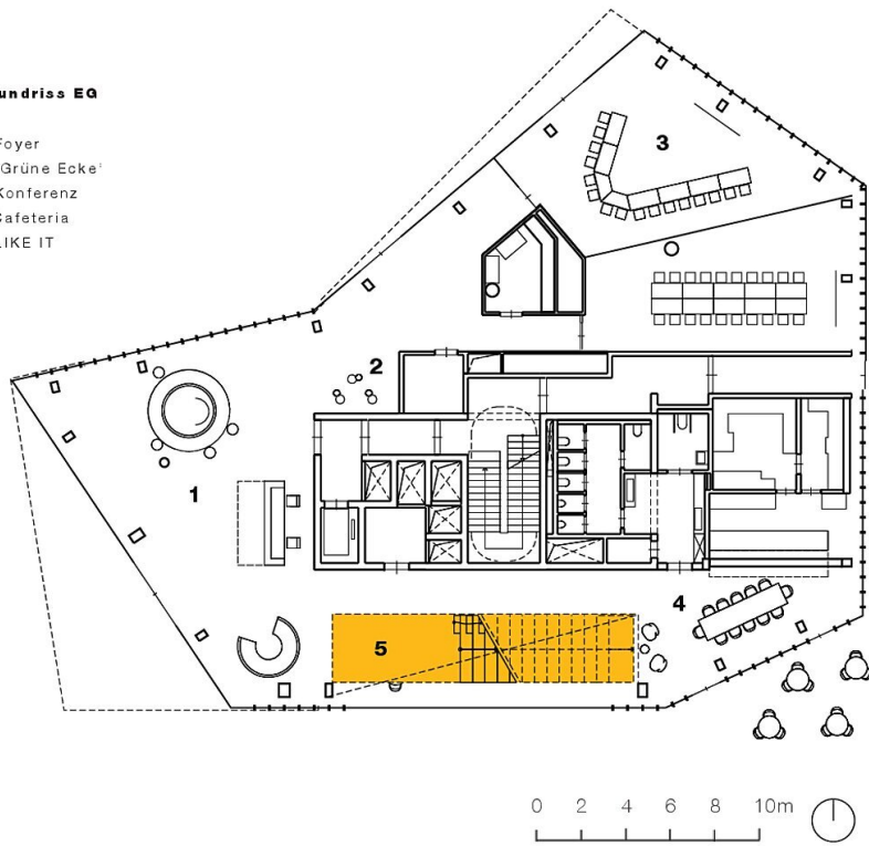
Grundriss EG
