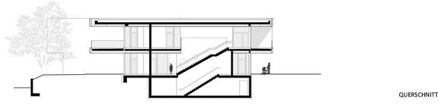
QUERSCHNITT
