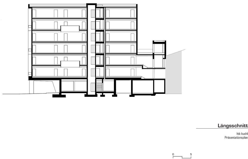
Längsschnitt
