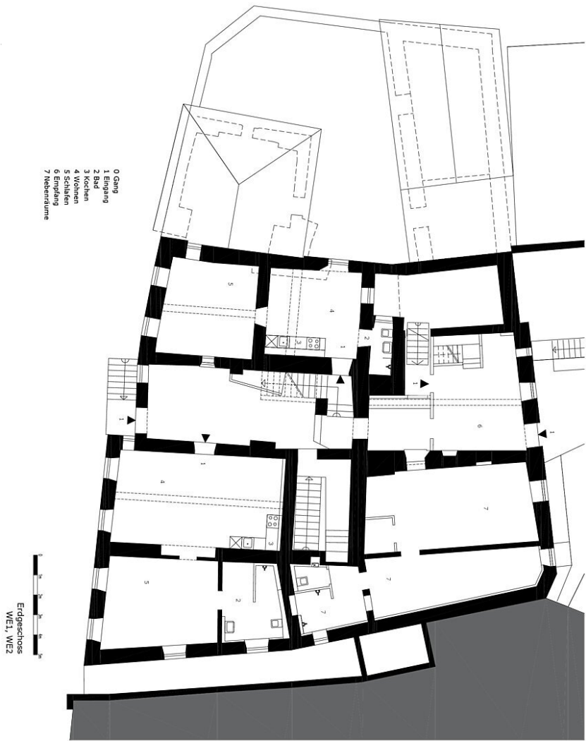
Grundriss EG
