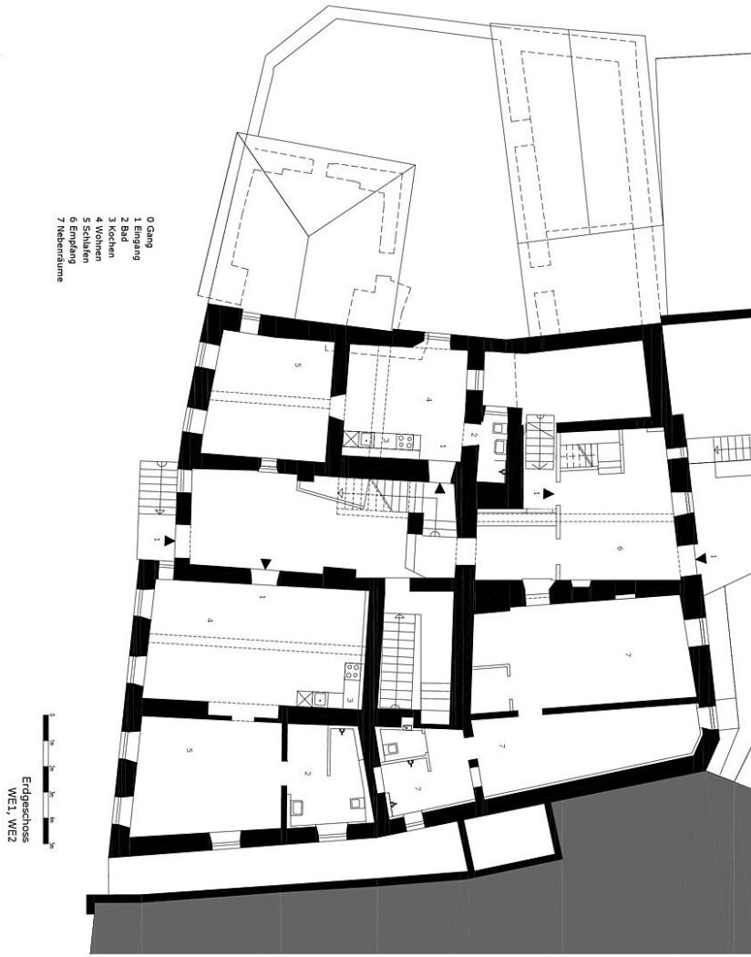
Grundriss EG
