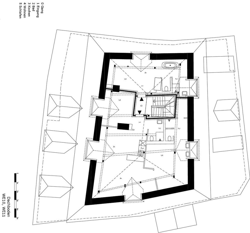
Dachboden
