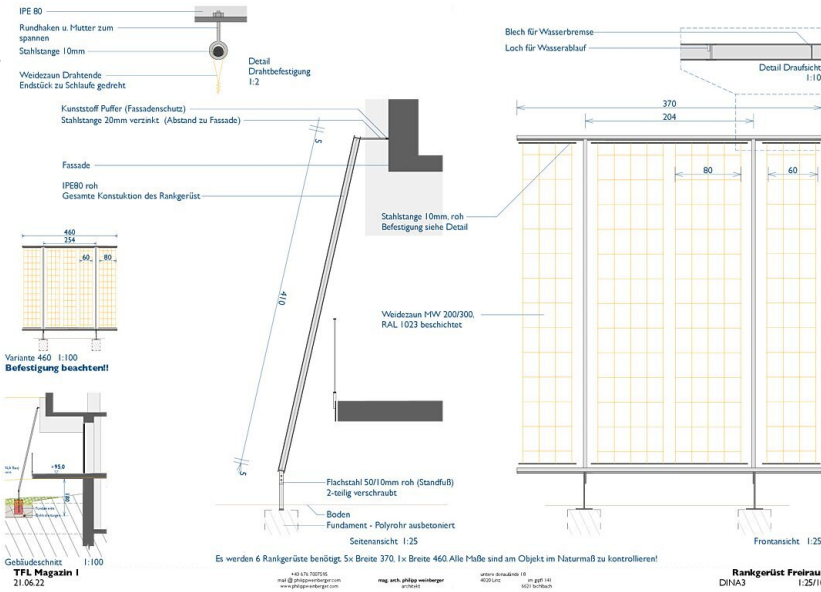
Rankerüst
