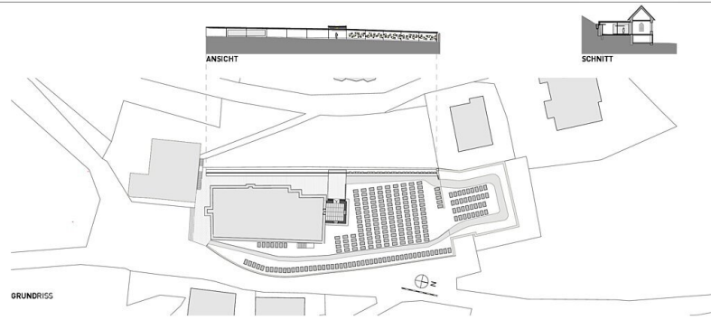
Grundriss, Ansicht, Schnitt
