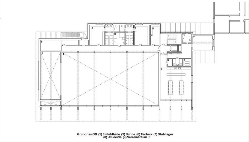
Grundriss OG
