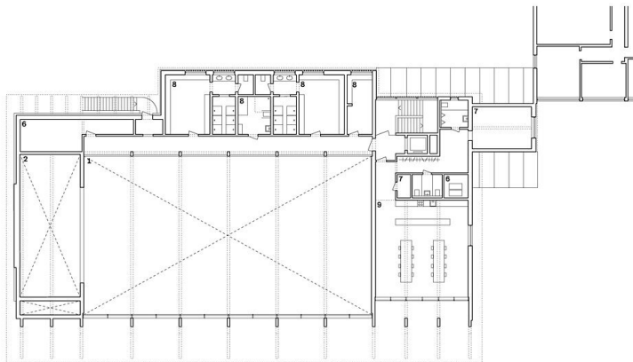
Grundriss OG (1) Einfeldhalle (2) Bühne (6) Technik (7) Stuhlilager (8) Umkleide (9) Verreinsraum ☉
